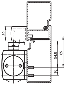
TS 5000 L. Dørbladmontasje på karmside med T-Stop Glideskinne BG
