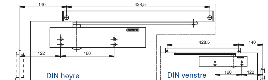
Montasje med dreielager på karmside
