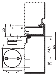
Montasje med dreielager på hengselside
