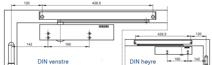
TS 5000 L. Dørbladmontasje på karmside med T-Stop Glideskinne BG
