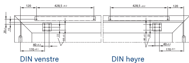
Montasje med dreielager på hengselside
