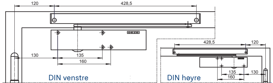
TS 5000. Dørbladmontasje på hengselside med T-Stop Glideskinne
