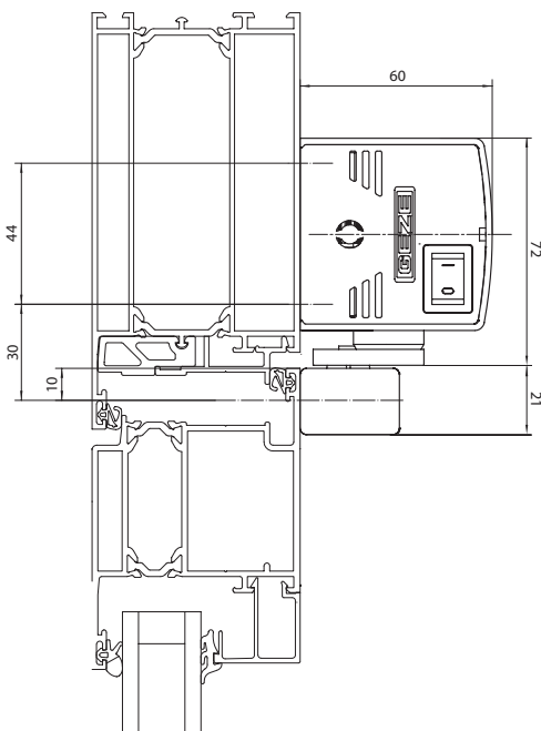
Montasje med glideskinne
