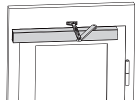
Montasje på dørlad med standard arm
